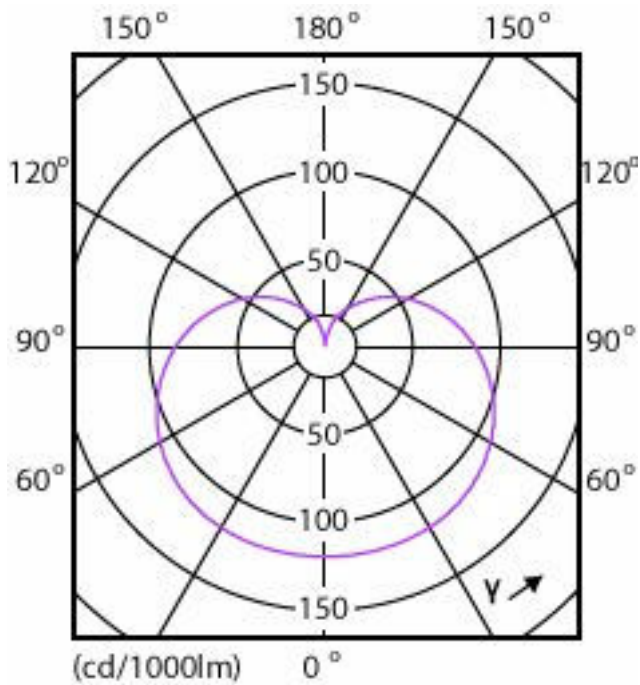
Light Distribution Diagram - 14A19/COR/950/FR/P/E26/DIM/T20 6/1CT
