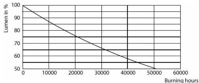
Lumen Maintenance Diagram - 14A19/COR/950/FR/P/E26/DIM/T20 6/1CT
