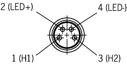
Ansicht auf Steckseite des Lesekopfs
