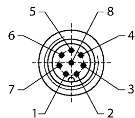
Ansicht auf Steckseite des Lesekopfs
