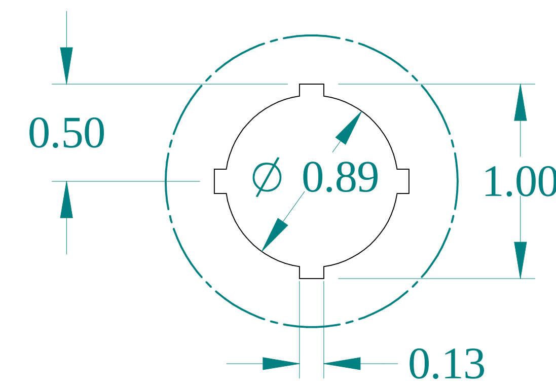
DETAIL Z TYP
