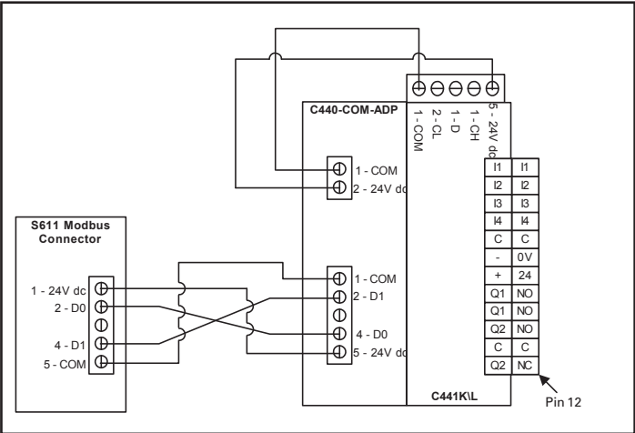
Figure 2. C441KL com module Wiring with S611 Softstarter
