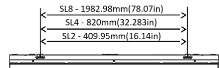
DISTANCE CENTRE À CENTRE DES SUPPORTS POUR MONTÉ EN SURFACE (SL2/SL4/SL8)
