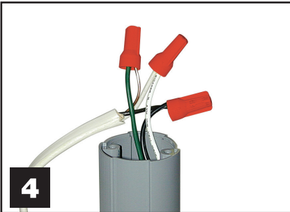
Figure 4 - Connect receptacle wires to NM Cable. Be sure to match wire color(s). Figure 4 - Connecter les fils de la prise au câble NM. Veiller à faire correspondre la/les couleur(s) des fils. Figura 4 - Conecte los cables del receptáculo al cable NM. Asegúrese de hacer coincidir los colores de los cables.
