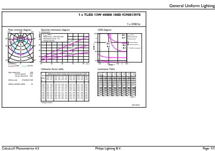
LEDtube 13W G13 2100lm
