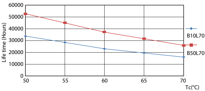
12W G13
